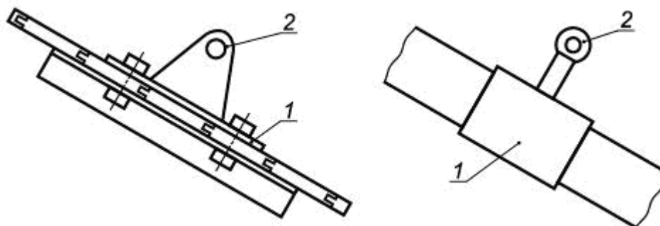
Рисунок 2 - Класс А2. Примеры структурных анкеров, предназначенных для крепления к наклонным крышам
