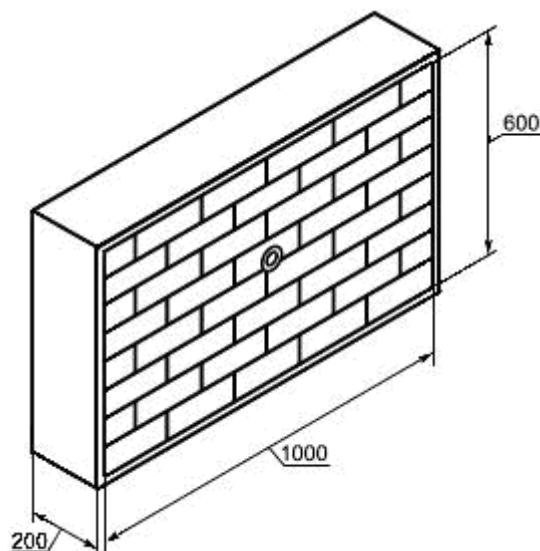
Рисунок 8 - Минимальный размер кирпичной кладки
