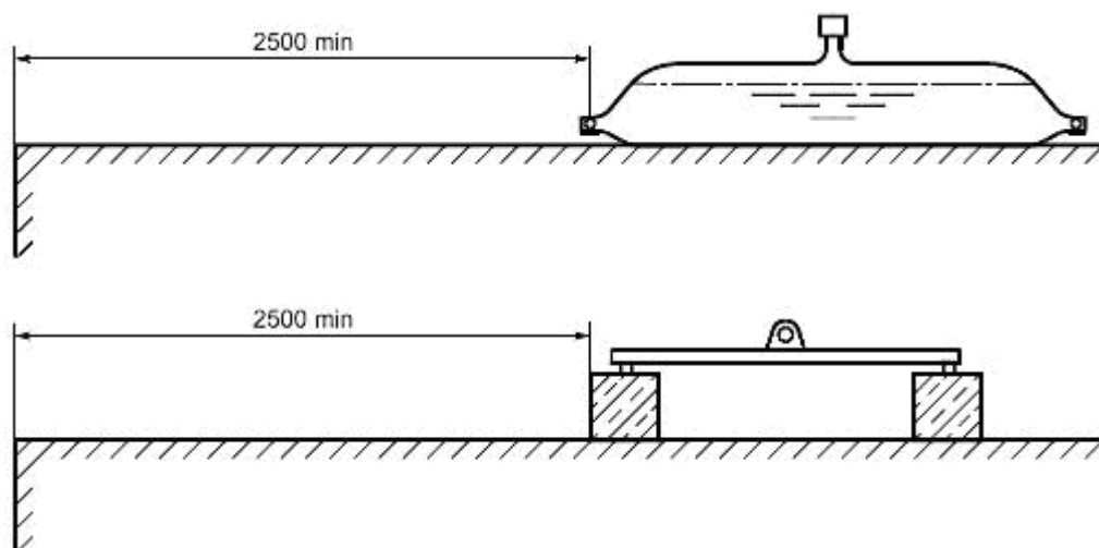
Рисунок 7 - Предельное расстояние до края крыши для анкерного устройства с противовесом
