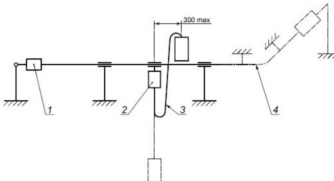
Рисунок 10 - Проверка динамической характеристики анкерных устройств класса С
