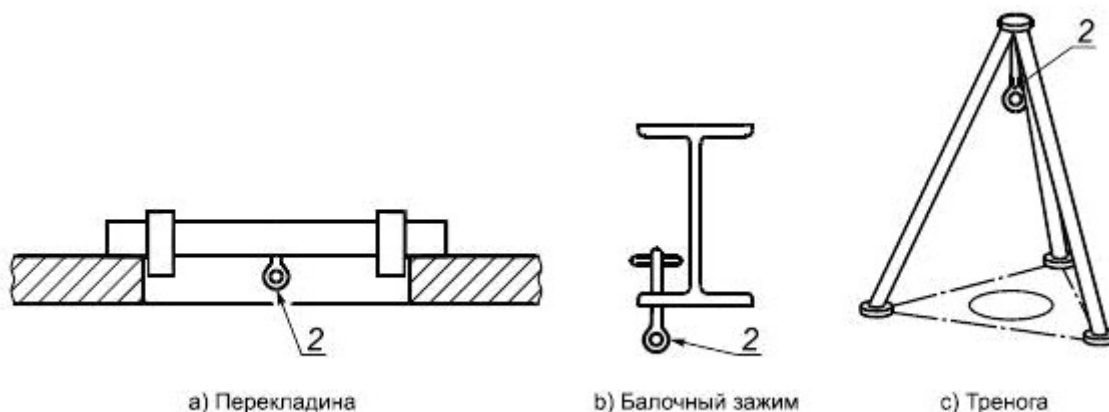
Рисунок 3 - Класс В. Примеры переносных временных анкерных устройств
