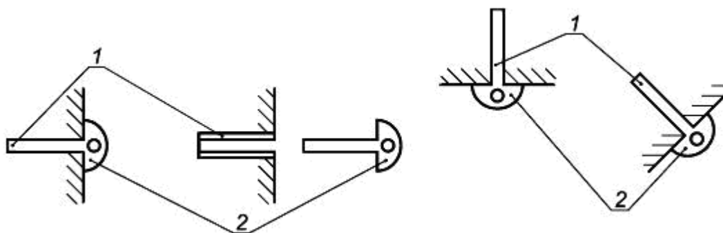
Рисунок 1 - Класс А1. Примеры структурных анкеров, предназначенных для крепления к вертикальным, горизонтальным и наклонным поверхностям
