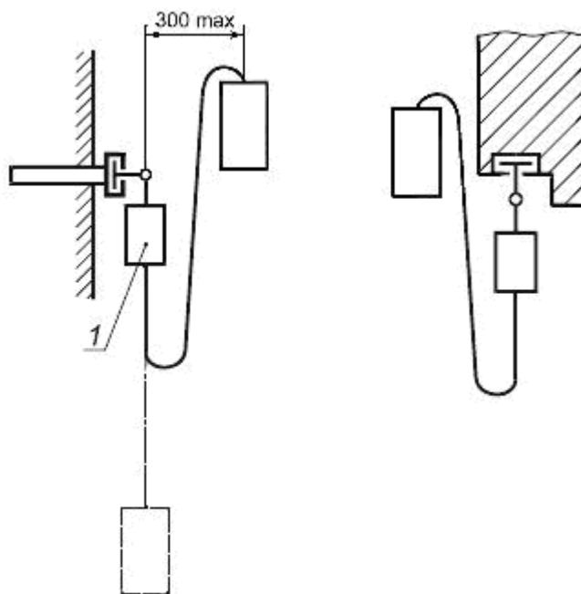
Рисунок 11 - Проверка динамической прочности на анкерных устройствах с жесткой горизонтальной направляющей
