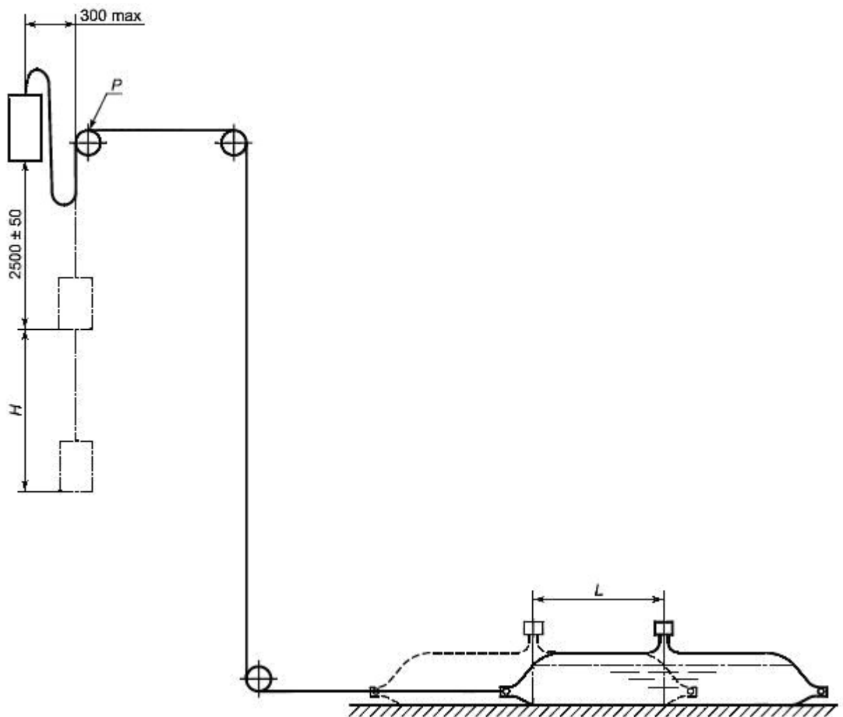
Рисунок 12 - Проверка динамической характеристики на устройствах анкерного крепления с противовесом
