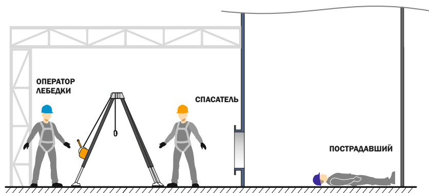
Рис. 11 Установка треноги.
