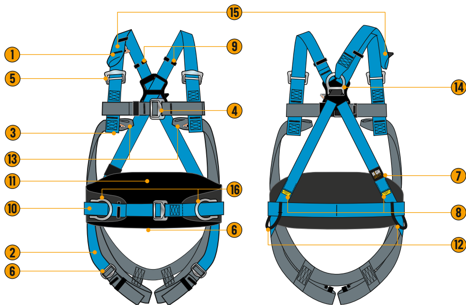
Рис. 2 Страховочная привязь BAZIS, арт. HS-50.
