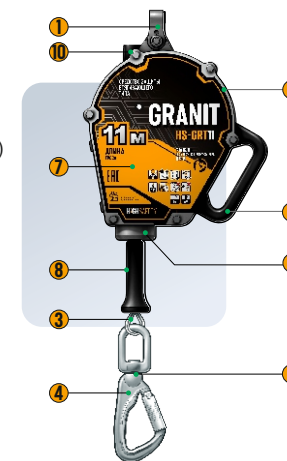
Рис. 1 Устройство СЗВТ GRANIT.
