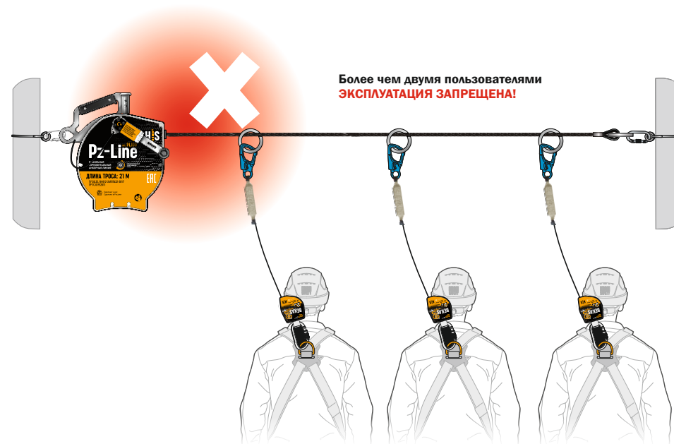
Рис. 12 Запрещено использовать анкерную линию более, чем двумя пользователями одновременно.
