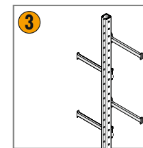
RVL500-12s/-24s/-36s/-48s/-60s ЖЁСТКАЯ АНКЕРНАЯ ЛИНИЯ (сегмент с интегрированными ступенями, длина 1,2/2,4/3,6/4,8/6 м)
