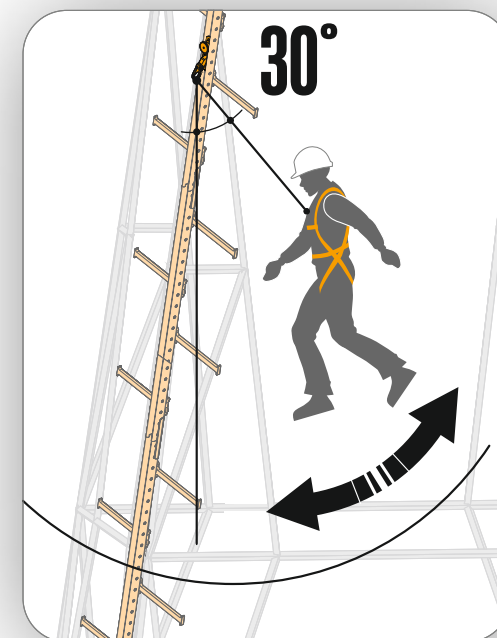
Рис. 5 Падение работника, сопровождающееся маятниковым движением.
