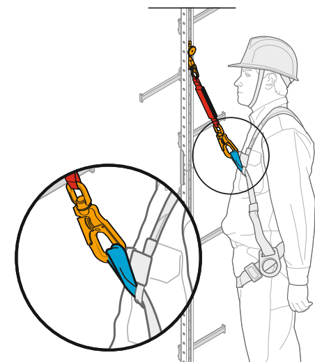
Рис. 6 Крепление соединительной подсистемы к анкерным точкам на привязи.
