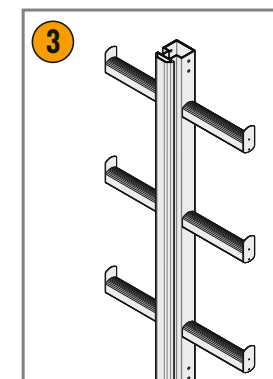
RVL20-01s/-02s/-03s ЖЁСТКАЯ АНКЕРНАЯ ЛИНИЯ (лестничный сегмент со ступенями, длина 1/2/3 м)
